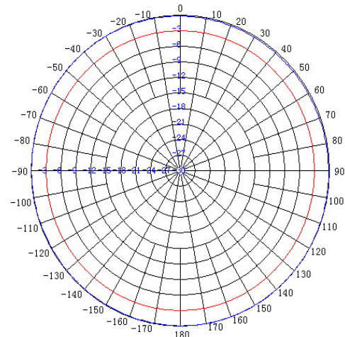
H-Plane
