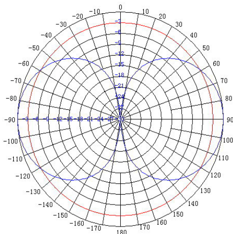
E-Plane
