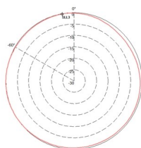
H-Plane Pattern
