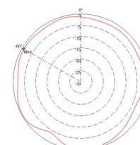
H-Plane Pattern
